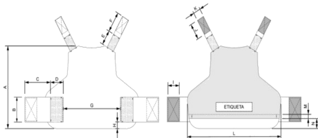
Figura 8 - Capa Dorsal – Dimensionais
