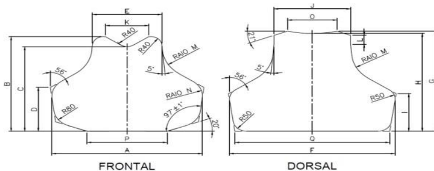
Figura 2 - Painéis Frontal e Dorsal, Modelo Feminino
