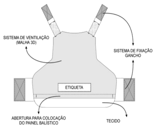
Figura 7 - Face Interna da Capa Dorsal
