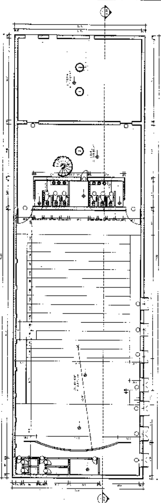
1) PLANTA BAIXA 1:100
